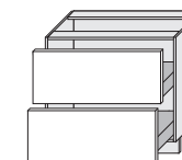
D2A/90 D2M/90 D2R/90 900/820/500
