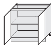
D11/90 900/820/500
