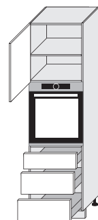
D14/RU/3A D14/RU/3M D14/RU/3R 600/2070/565
